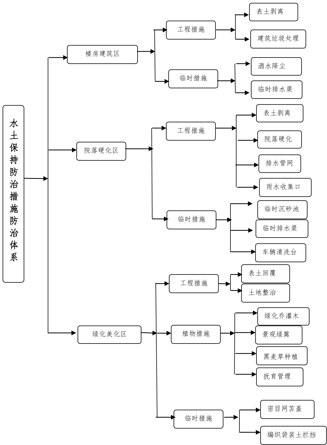
5-3 水土保持措施防治体系框图
