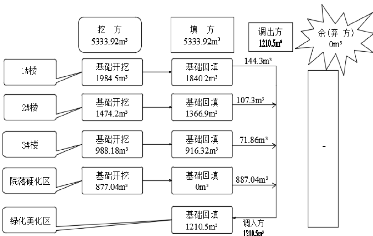
图 2-6 土石方流向框图
