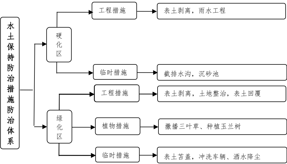
图 6-1 本项目水土流失防治措施体系框图
