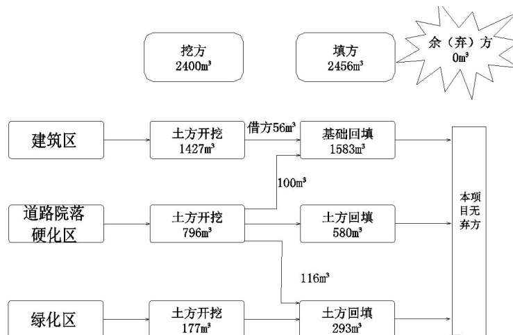
图 2-1 土石方平衡及流向图 （单位: m 3 ）
