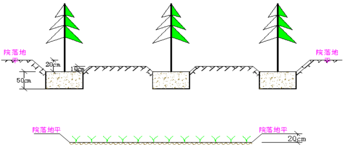
图 5-7 树池及草坪低位绿地结构设计图
