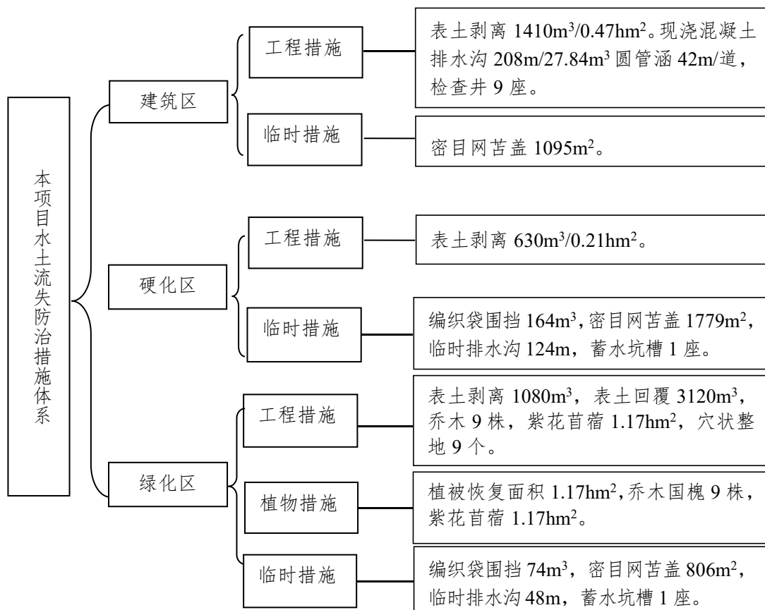
图 5-1 项目水土流失防治措施体系框图
