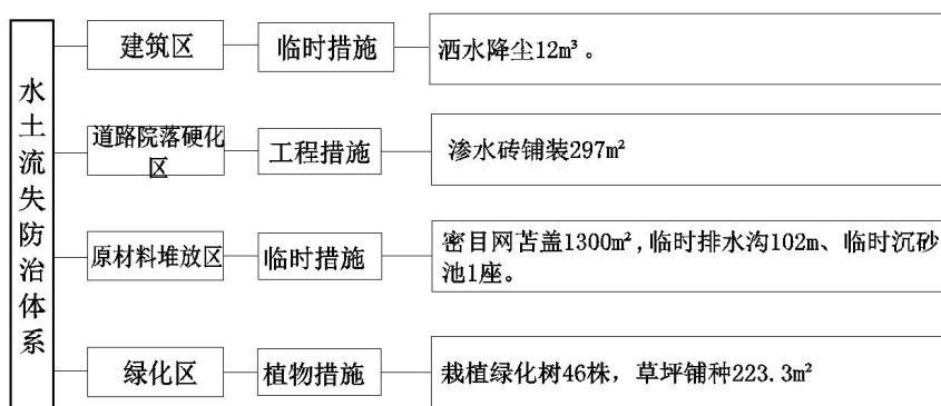
图 5-1 水土保持工程防治体系框图
