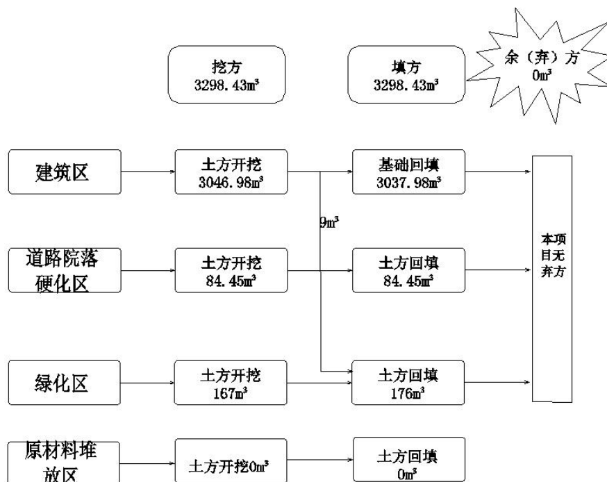
图 2-1 土石方平衡及流向图 (单位: \text{m}^3 )
