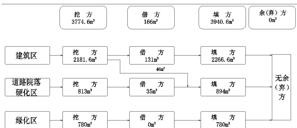
图 2-1 土石方平衡及流向图 (单位: \text{m}^3 )
