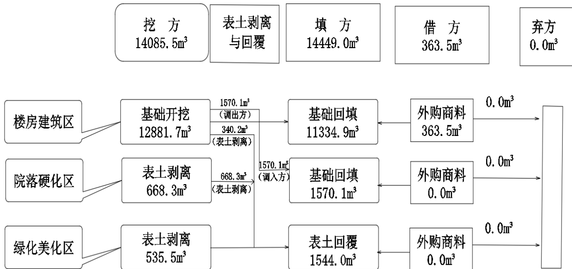
图 2-6 土石方流向框图
