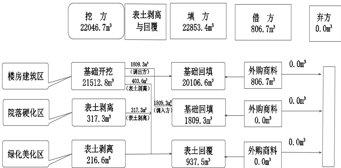
图 2-5 土石方流向框图
