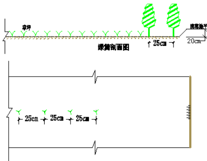
图 5-9 绿篱栽植图
