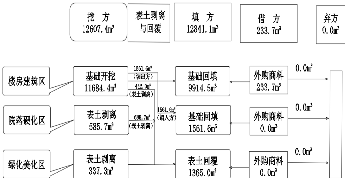
图 2-6 土石方流向框图
