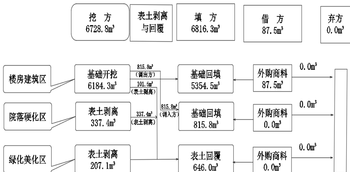
图 2-7 土石方流向框图
