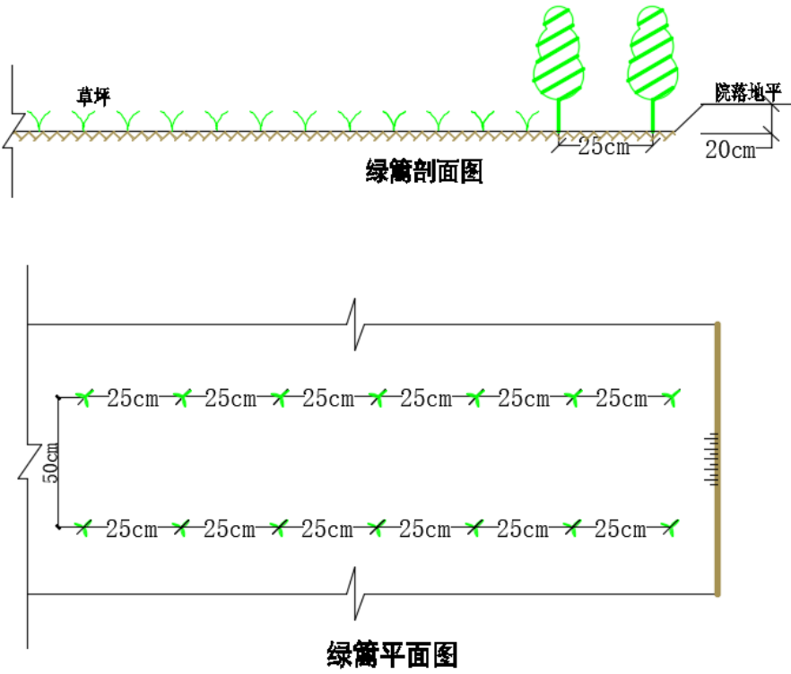
图 5-9 绿篱栽植图
