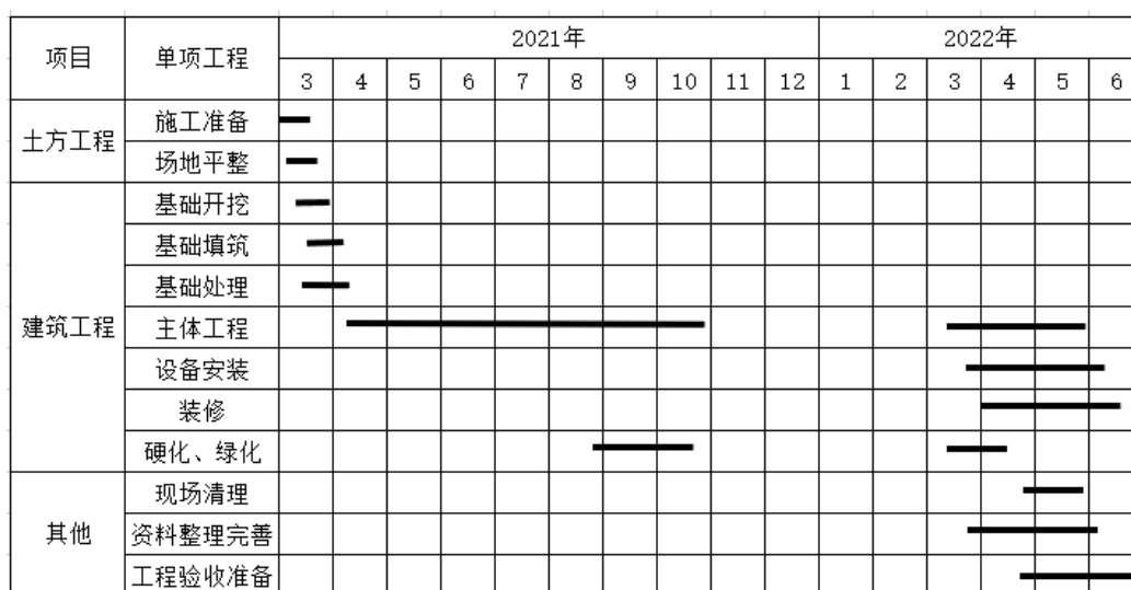
图 2-8 主体工程施工进度横道图
