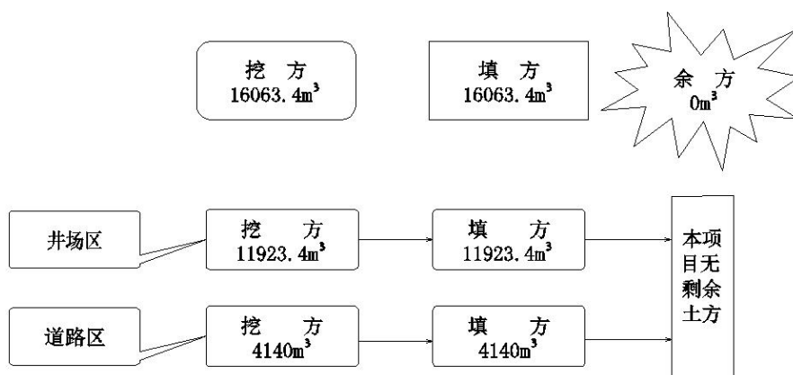
图 2-1 土石方平衡及流向图 (单位: \text{m}^3 )
