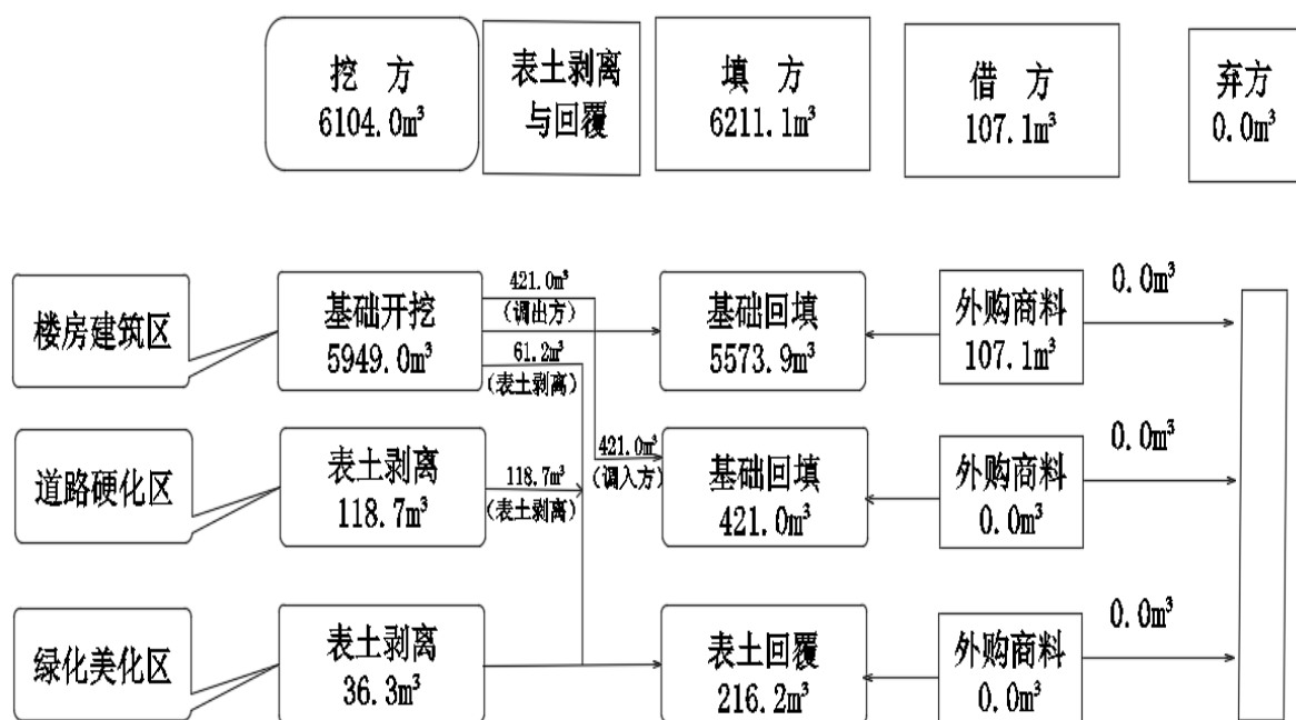
图 2-6 土石方流向框图
