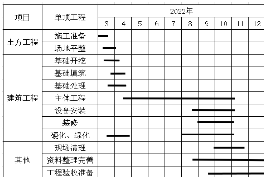
图 2-7 主体工程施工进度横道图
