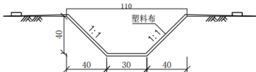
图 5-7 临时排水沟典型设计
