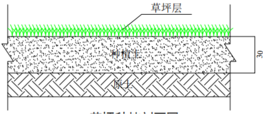
图 5-14 种草典型设计
