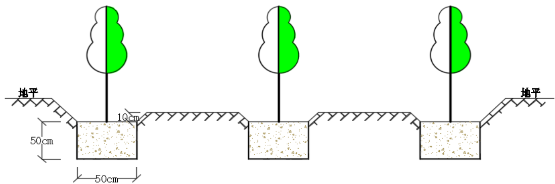
图 5-17 灌木栽植典型设计
