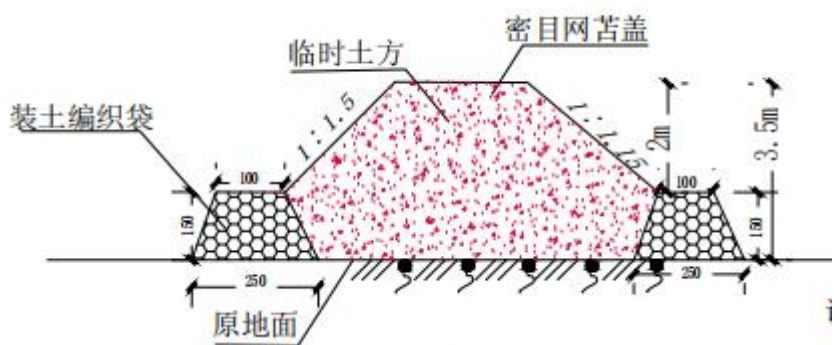
图 5-18 编织袋装土拦挡典型设计
