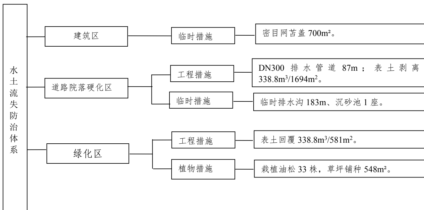
图 5-1 水土保持工程防治体系框图
