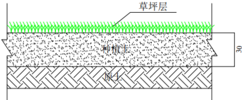
图 5-14 种草典型设计
