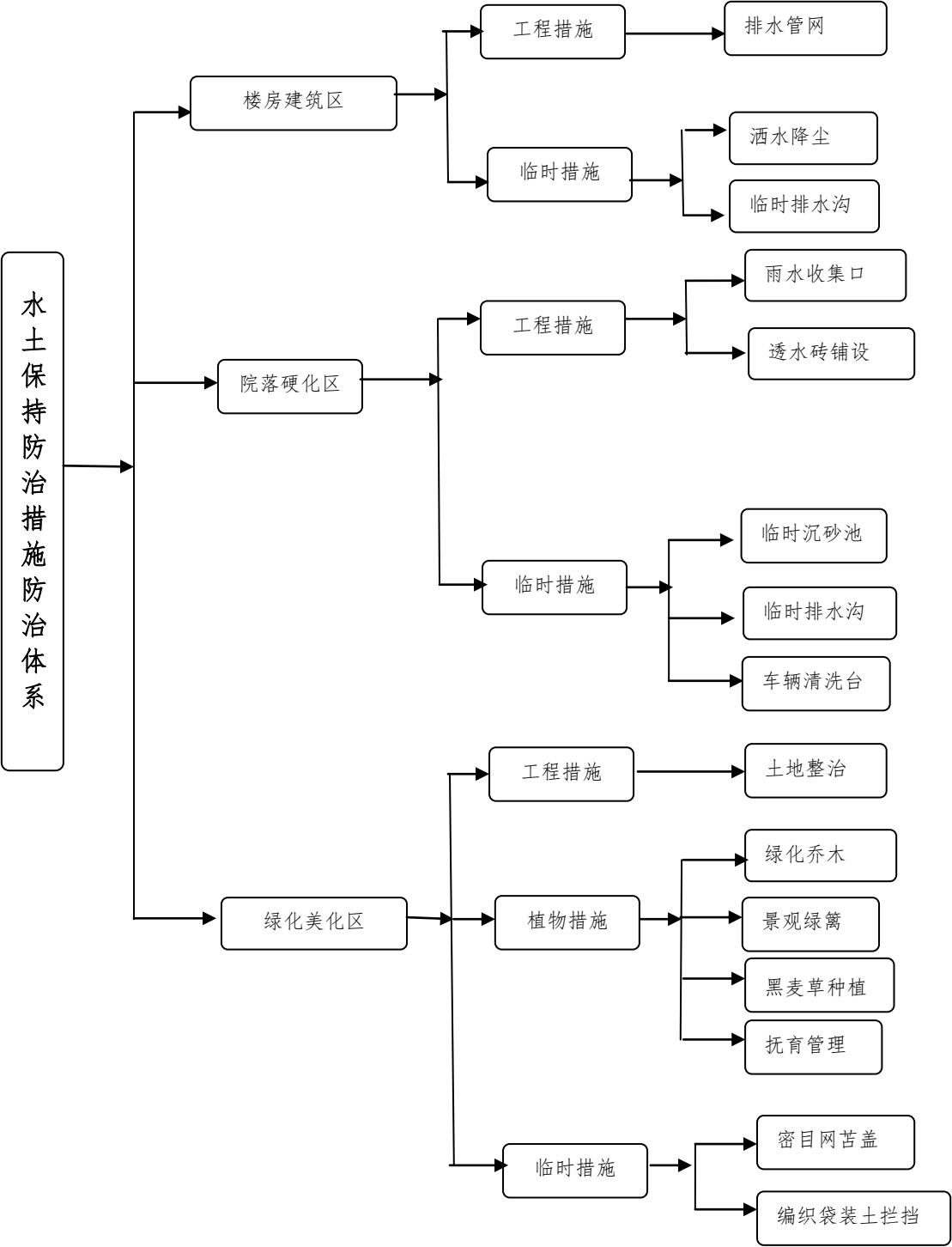
图 5-3 水土保持措施防治体系框图
