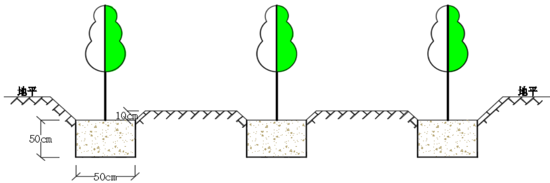
图 5-17 灌木栽植典型设计
