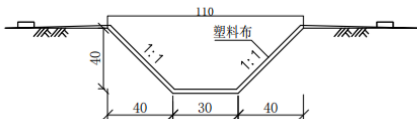
图 5-16 临时排水沟典型设计图
