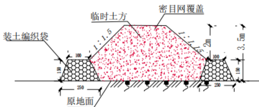
图 5-18 编织袋装土拦挡典型设计图
