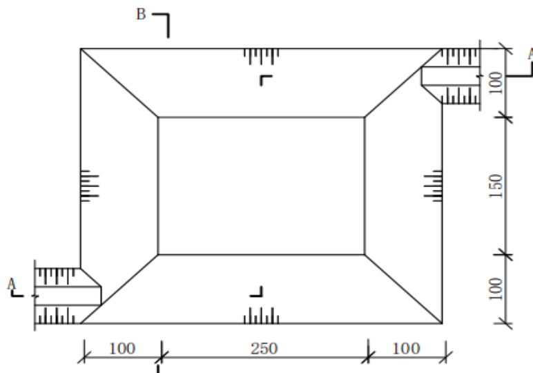
图 5-17 临时沉砂池典型设计图
