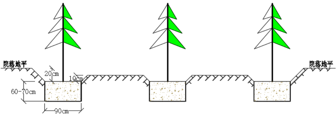
图 5-10 乔木栽植典型设计
