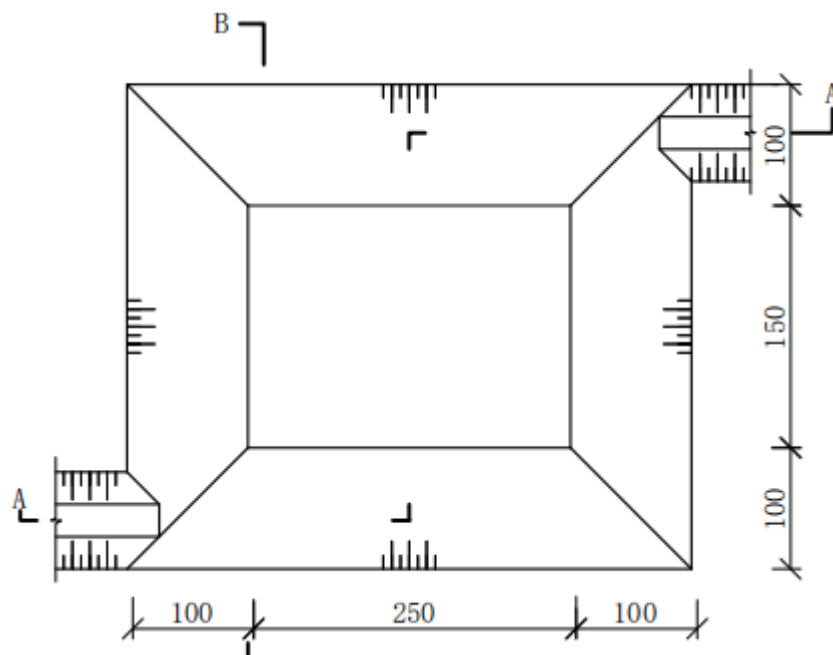
图 5-8 临时沉砂池典型设计
