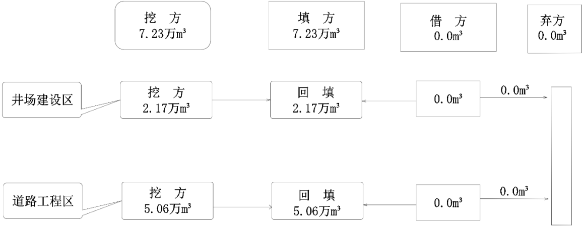
图 2-2 土石方流向框图
